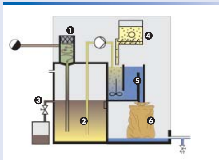
Funcionamiento BEKOSPLIT® 11
