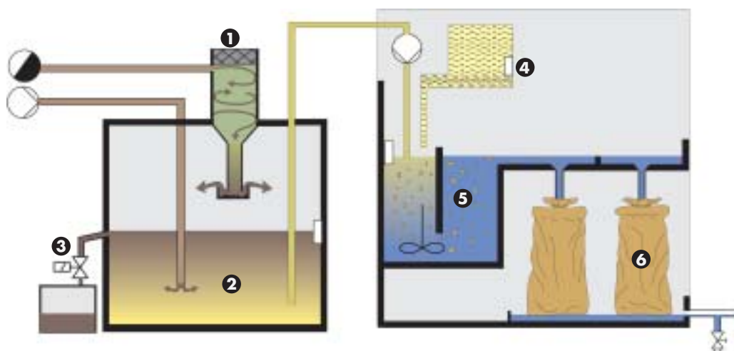
Funcionamiento BEKOSPLIT® 12-16
